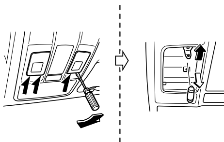
バニティミラーランプ
