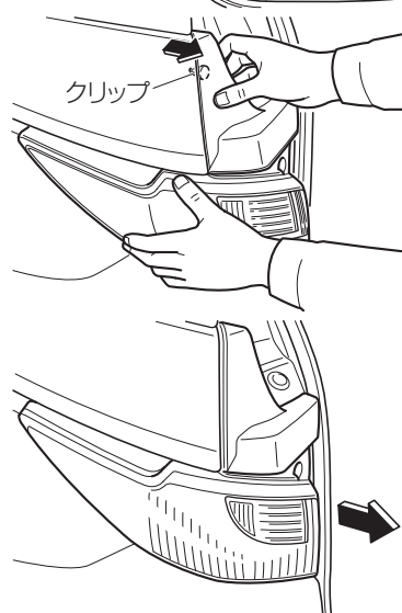
制動灯/尾灯
