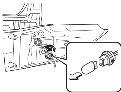
制動灯/尾灯
