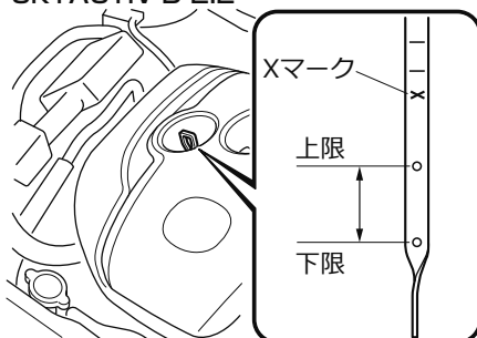
SKYACTIV-D 2.2
