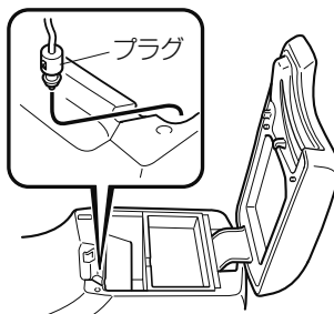
電動パーキングブレーキ (EPB) 非装備車
