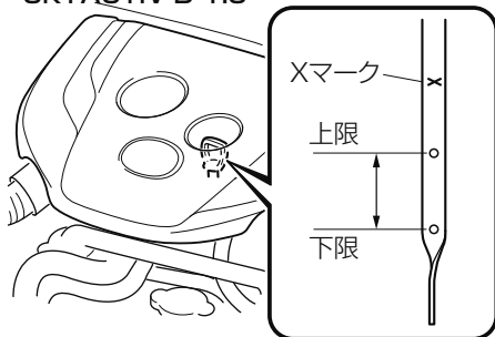
SKYACTIV-D 1.5
