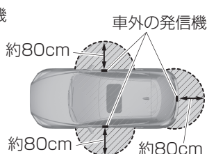
ハッチバック（施錠）
