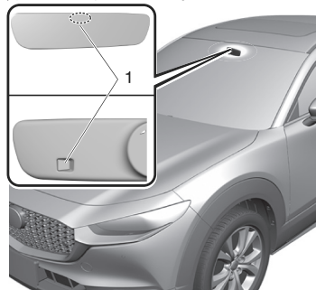
1 センサー
