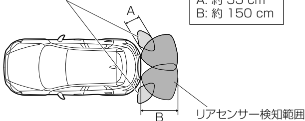
リアコーナーセンサー検知範囲
