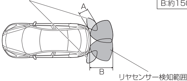
リヤコーナーセンサー検知範囲
