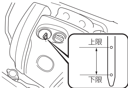
SKYACTIV-G 2.0, SKYACTIV-G 2.5
