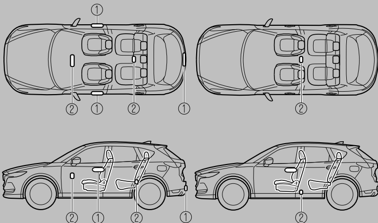
①車外のアンテナ ②車内のアンテナ
