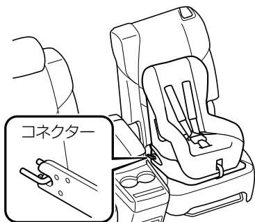
ロアアンカレッジ
