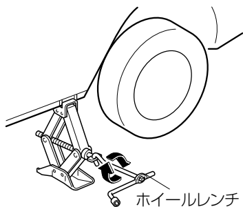
ホイールレンチ
