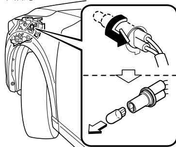
車幅灯
