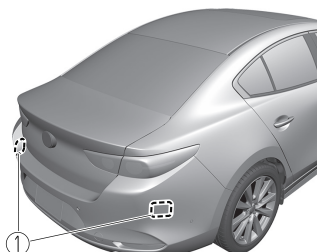
1. リアサイドレーダーセンサー ファストバック
