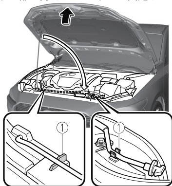
1. クリップ
