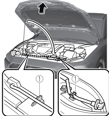
1. クリップ
