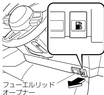
フューエルリッド
