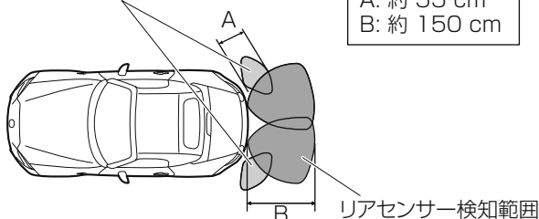
リアコーナーセンサー検知範囲
