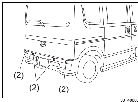
(2) 超音波センサー
