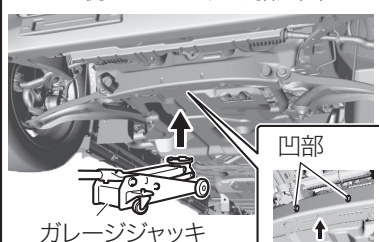
フロント側ガレージジャッキ指定位置
