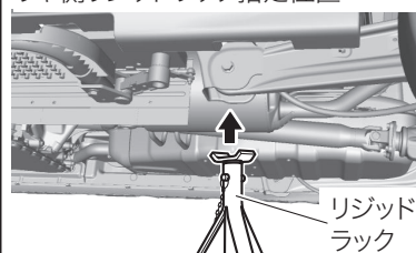
リヤ側リジッドラック指定位置
