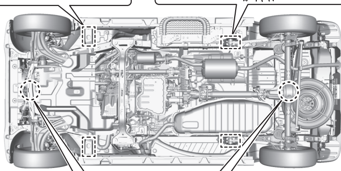
フロント側ガレージジャッキ指定位置
