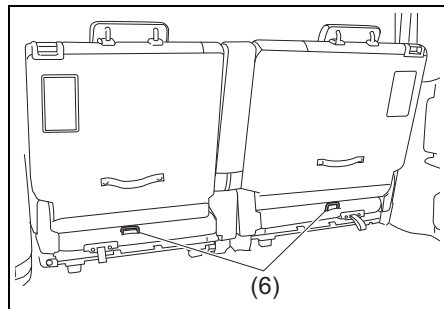
(6) テザーアンカー
