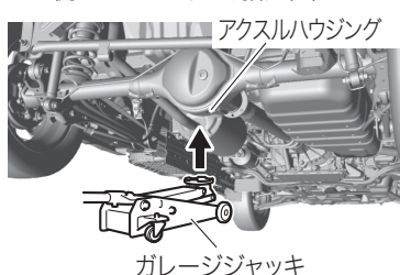
リヤ側ガレージジャッキ指定位置
