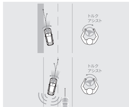
車線からの逸脱回避を支援する 運転支援機能 緊急時車線維持支援 [側方危険回避アシスト機能 & ロードキープアシスト機能] (ELK) ※6※7※8
