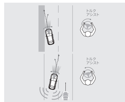
車線からの逸脱回避を支援する 緊急時車線維持支援 [側方危険回避アシスト機能 / ロードキープアシスト機能] (ELK) ※2※3※6
